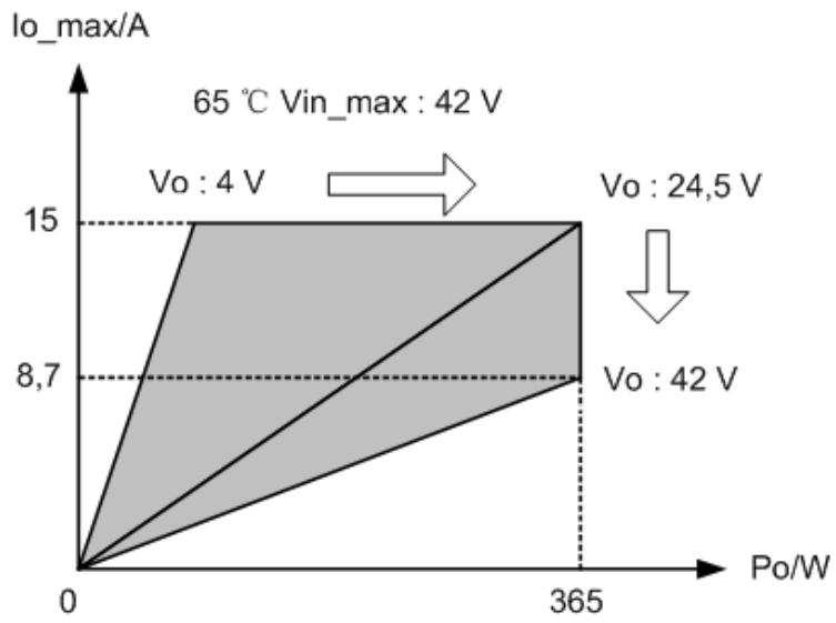
Figure A-3 Courbe de relation I_{o\_max} - P_o ( 65^\circ\text{C} , V_{in\_max} = 42\text{ V} )
