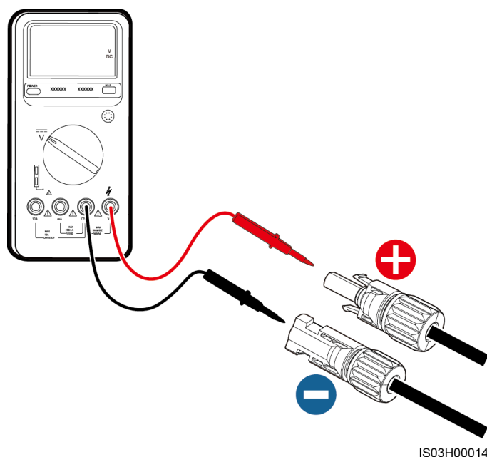
Figure 3-1 Mesure de la tension de sortie du SUN2000P
