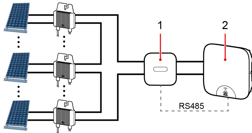
Figure 2-3 SUN2000P configurés pour tous les modules photovoltaïques
