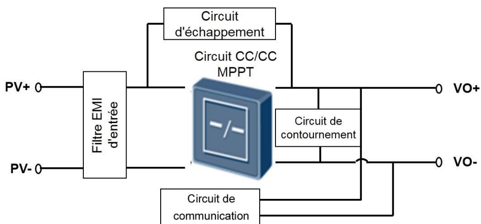
Figure 2-2 Schéma conceptuel
