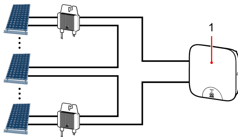
Figure 2-4 SUN2000P configurés pour les modules photovoltaïques ombragés
