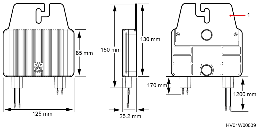
Figure 2-7 Dimensions du produit
