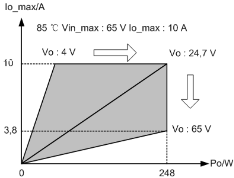
Figure A-5 Courbe de relation I_{o\_max} - P_o ( 85^\circ\text{C} , V_{in\_max} = 65\text{ V} , I_{o\_max} = 10\text{ A} )
