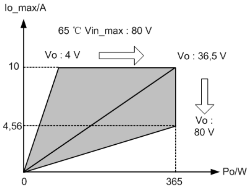
Figure A-4 Courbe de relation I_{o\_max} - P_o ( 65^\circ\text{C} , V_{in\_max} = 80\text{ V} )
